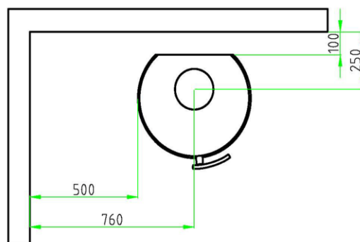
Mått till brännbart, placering mot vägg
